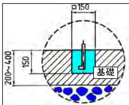
φ12×6時のアンカーボルト使用の場合
