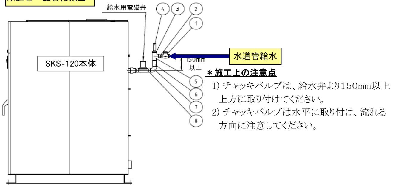
水道管へ配管接続図
