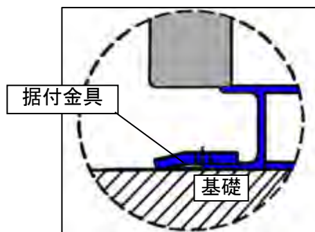
据付用金具使用の場合
