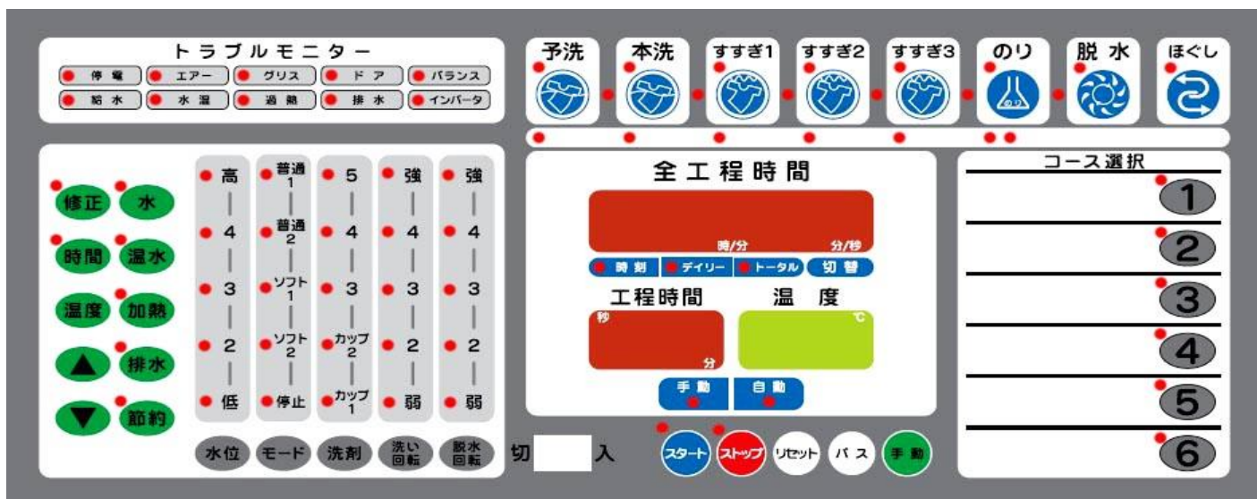
7-1 ドラム回転を行う場合(モードー普通, 回転ー5)
