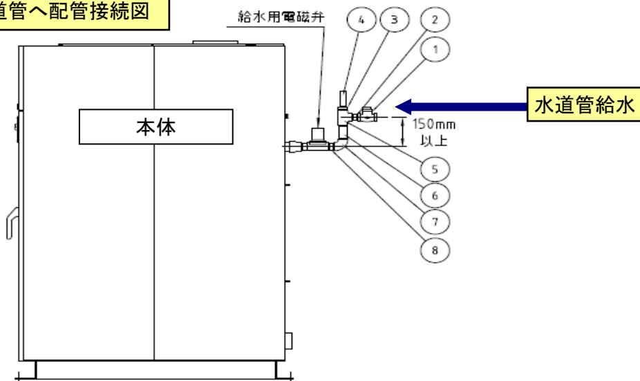
水道管へ配管接続図
