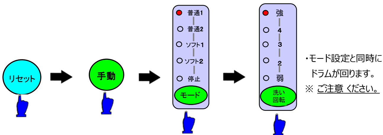
7-1 ドラム回転を行う場合(モードー普通, 回転ー5)
